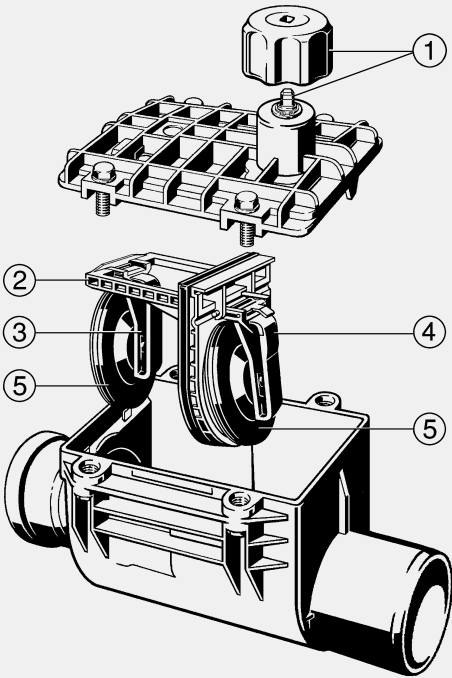
Grundfix B alkatrészcsomag modellszám 4986.39
