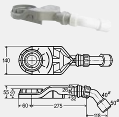
Advantix szifon (felújításokhoz) - a következőkhöz: Advantix saroklefolyók átalakítása 66 mm beépítési magasságra - az alábbiakhoz használható: Advantix saroklefolyó modell 4972.80, 4972.81, 4972.82, 4972.83 Kialakítás/felszereltség csatlakozóvezeték tisztítási lehetősége, kivehető szűrőbetét műszaki adatok zárvízmagasság 25 mm lefolyási teljesítmény torlasztási magasság 10 mm 0,4 l/s lefolyási teljesítmény torlasztási magasság 20 mm 0,45 l/s lefolyási teljesítmény az MSZ EN 1253 szerint modellszám 4980.65
