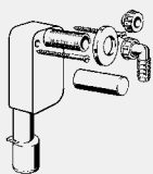
Szifon - a következőkhöz: falba építés, mosó- vagy mosogatógép szennyvíztömlő - műanyag Kialakítás/felszereltség függőleges lefolyócső, rögzítőcsavarok, védősapka menethez, 90°-os tömlőcsavarzat, zárókupak, nemesacél rozetta DIN 19541 minőségellenőrzött modellszám 5635.7
