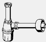
Búraszifon - műanyag Kialakítás/felszereltség Ø 50 tányér modellszám 5725
