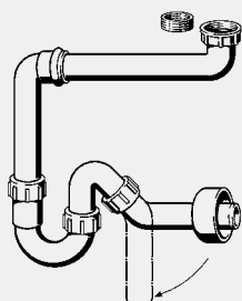
Csőszifon - műanyag Kialakítás/felszereltség 45°-os lefolyóív modellszám 97512
