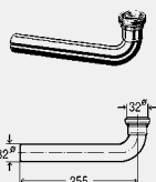
90°-os lefolyóív - krómozott sárgaréz modellszám 5622.2
