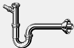
Csőszifon Plus szifon - krómozott sárgaréz Kialakítás/felszereltség G 3/4-es tömlőcsavarzat, lezárólemez, 200 mm-es állítócső, 220 mm-es lefolyóív DIN EN 274 minőségellenőrzött modellszám 5611.6
